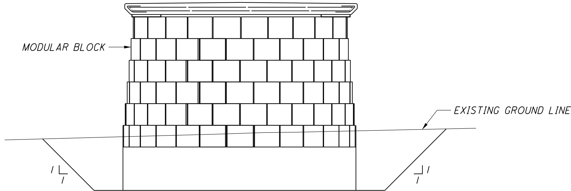
ELEVATION SCALE: 1/4" = 1'-0"
