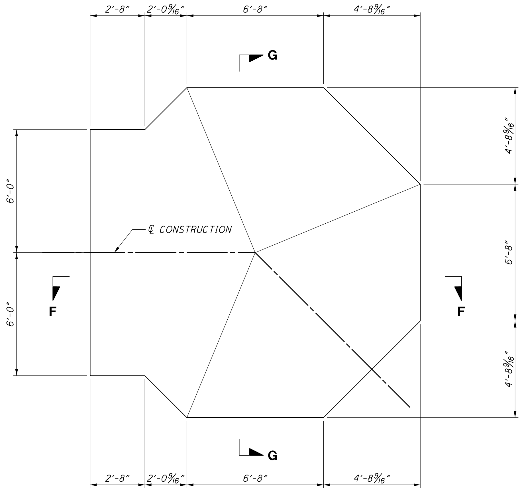
SLAB PLAN SCALE: 3/8" = 1'-0"
