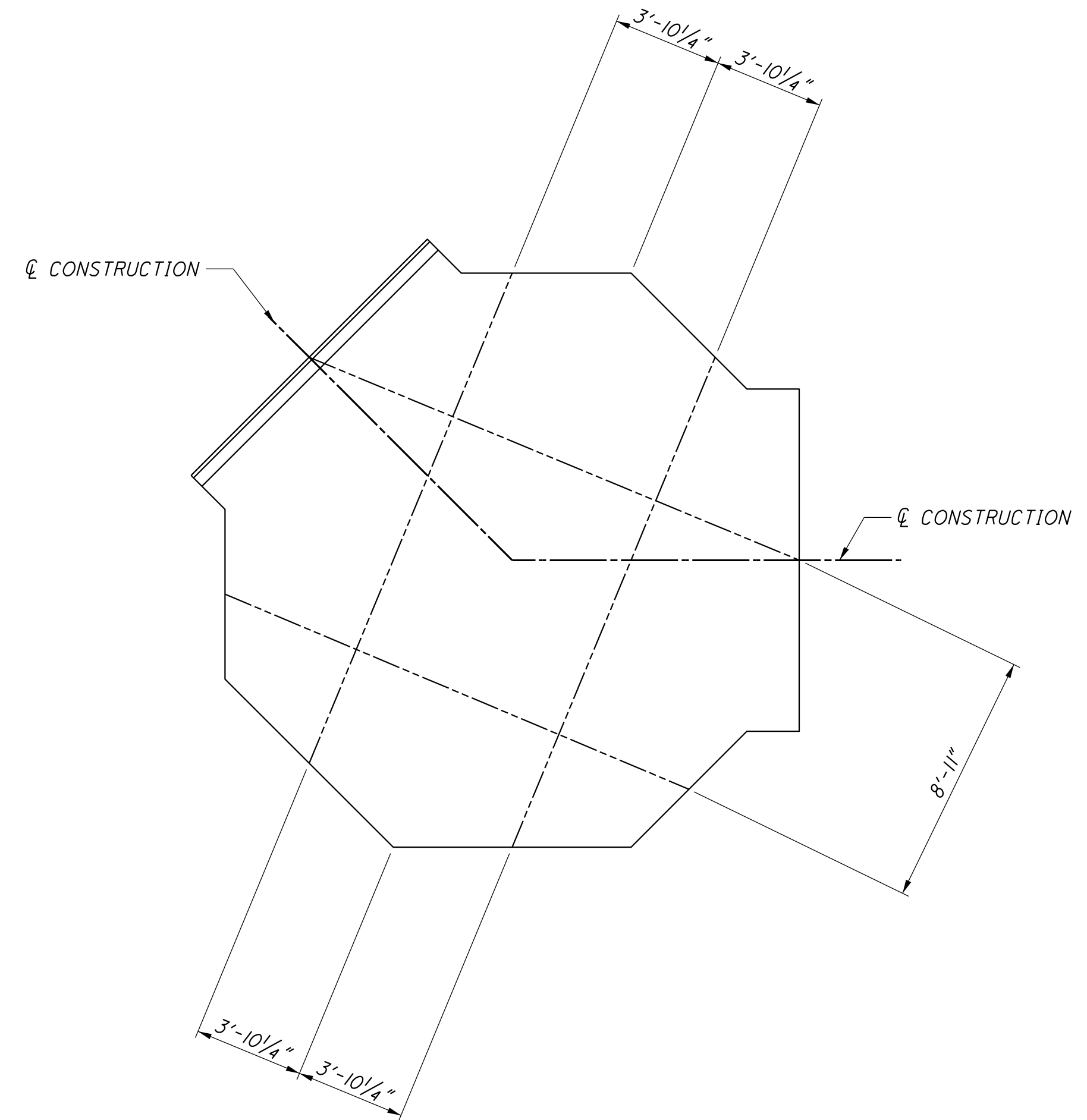
SAWCUT PLAN SCALE: \frac{1}{4}" = 1'-0"
