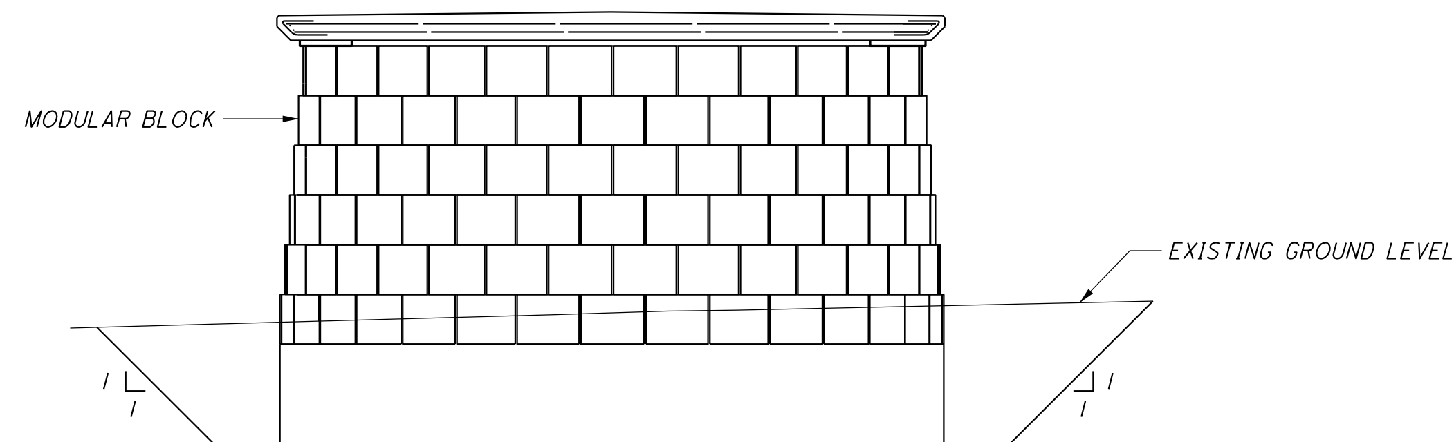
ELEVATION SCALE: 1/4" = 1'-0"
