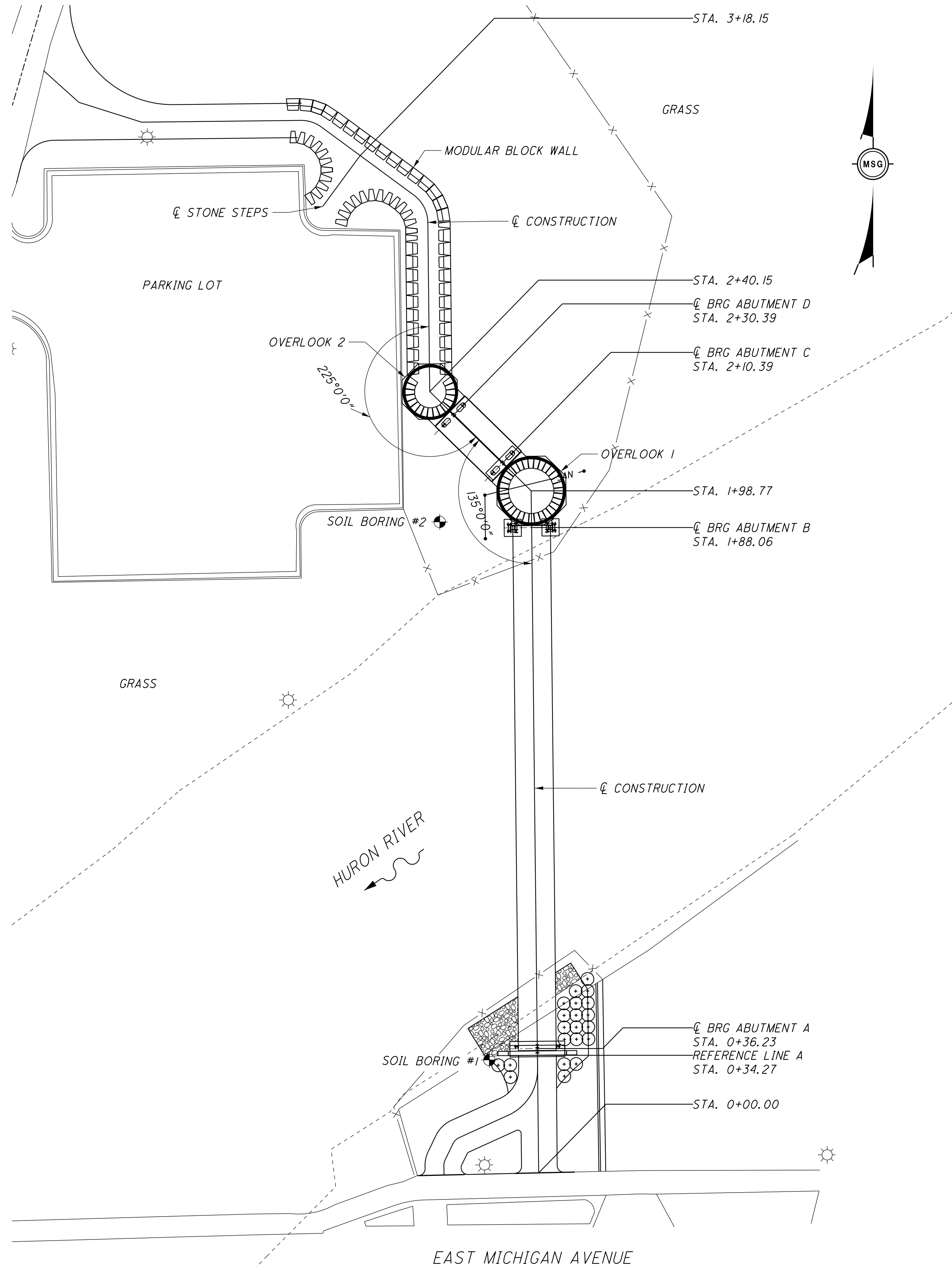
PLAN SCALE: 1" = 20'-0"
